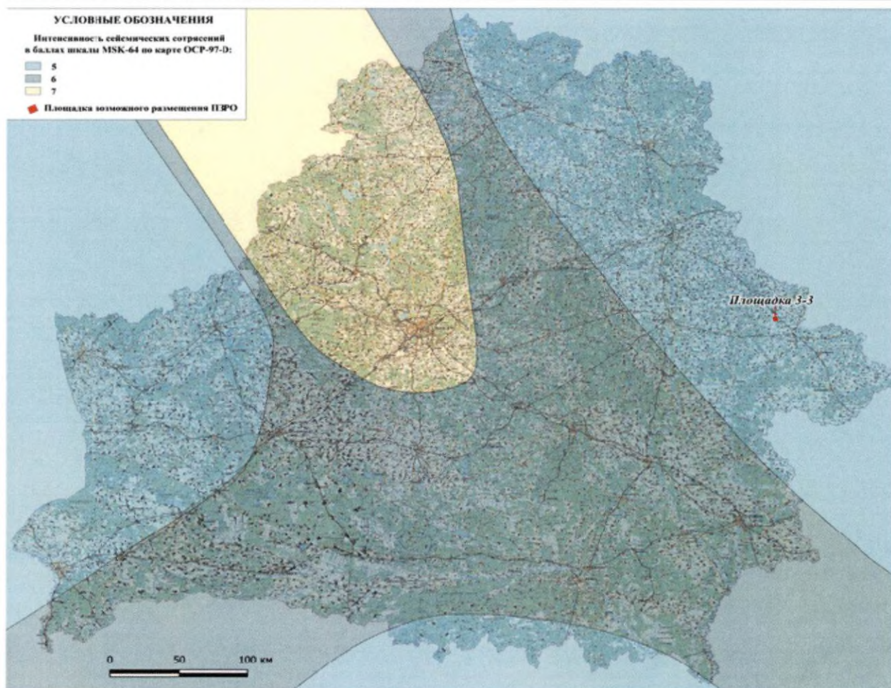
Рисунок 5.10 – Фрагмент Карты ОСР-97D с указанием положения альтернативной площадки 3-3 размещения ПЗРО
