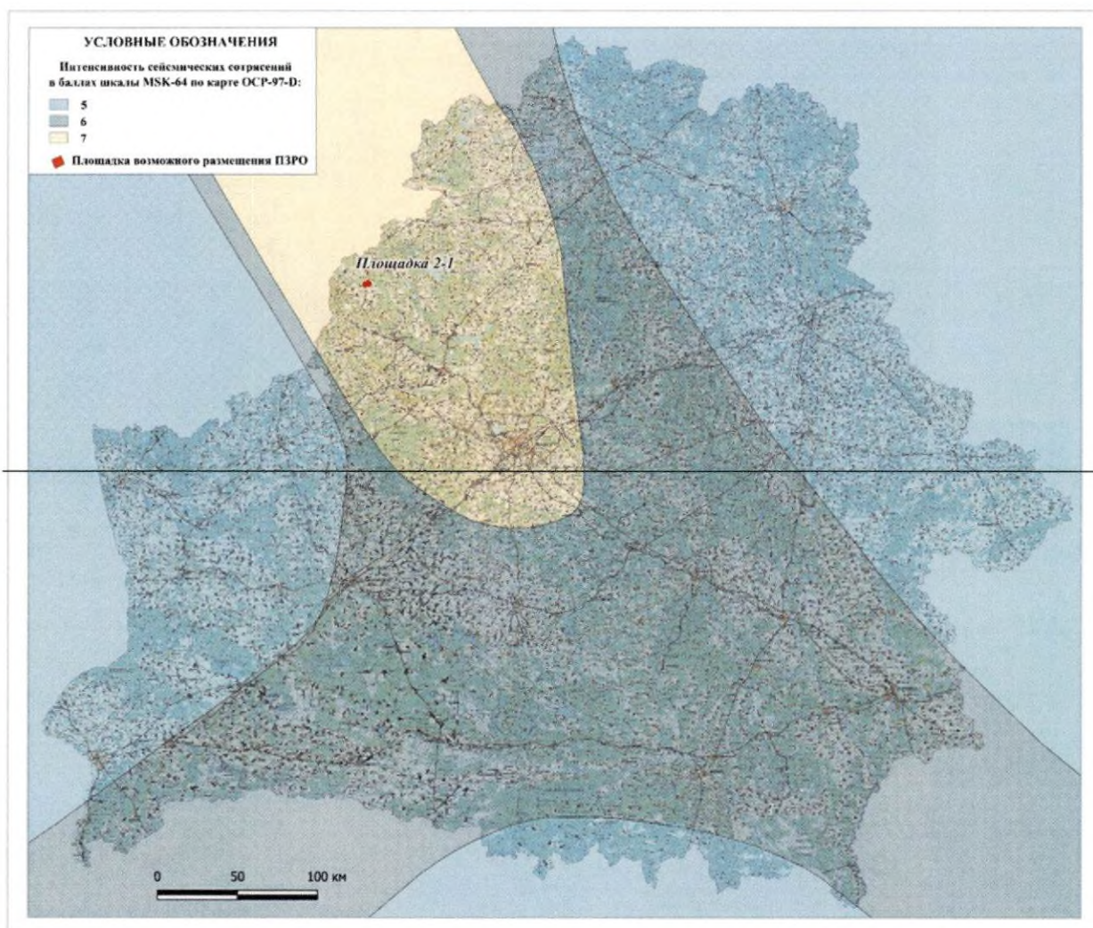
Рисунок 5.7 – Фрагмент Карты ОСР-97Д с указанием положения площадки 2-1 размещения ПЗРО
