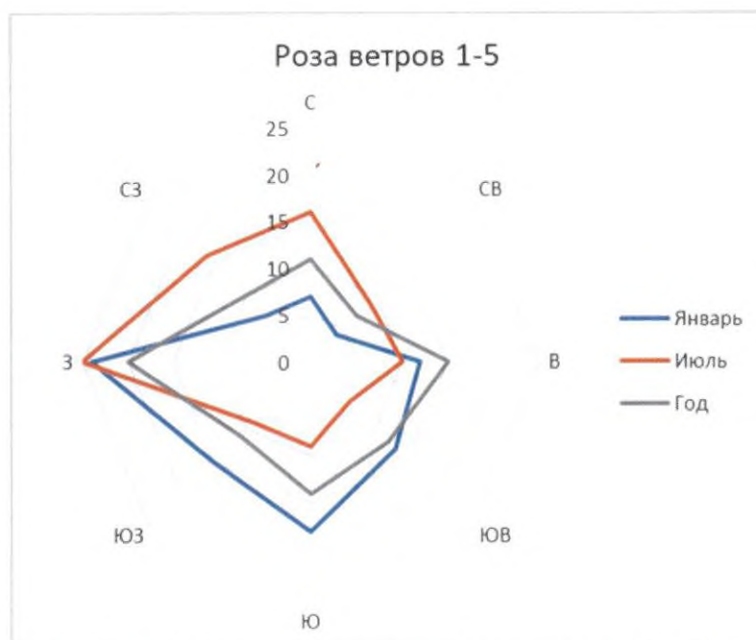
Рисунок 5.3 – Среднегодовая роза ветров
